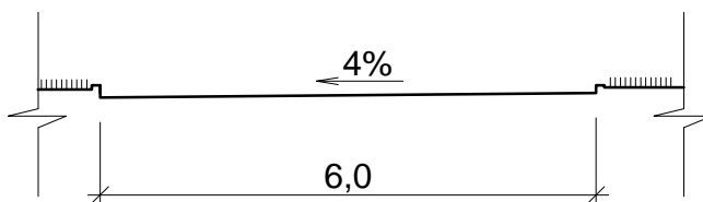
Поперечний профіль проїзду (1:100) Розріз 1-1.
